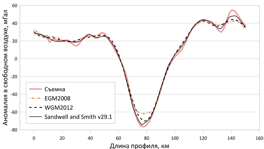
Рис. 9. Графики АСТ по данным морской гравиметрической съемки и моделей ГПЗ в градиентной области (Срединно-океанический хребет, Индийский океан)
