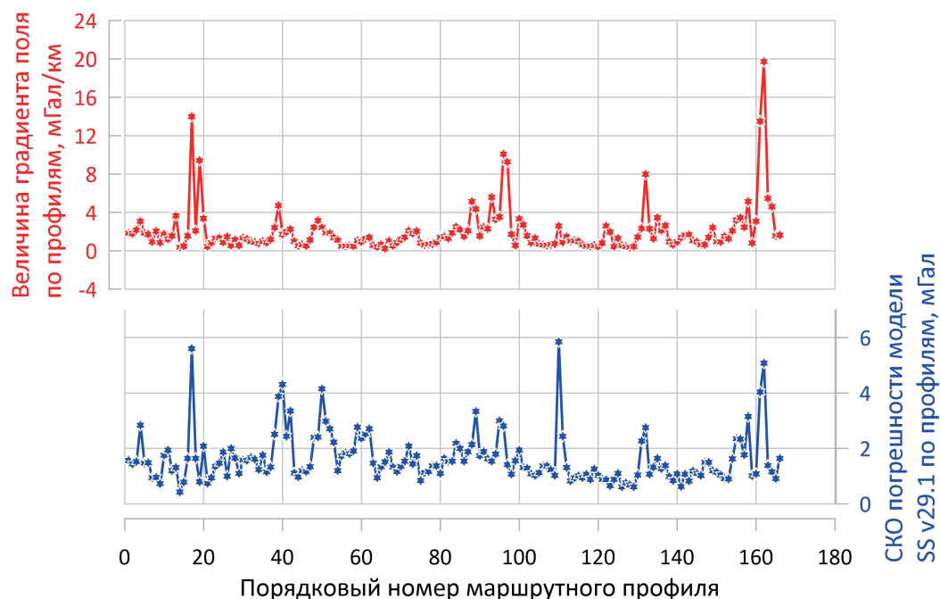
Рис. 6. Графики изменения градиента и СКО модельных АСТ Sandwell and Smith v29.1 по 166 протяженным маршрутным профилям в основных акваториях Мирового океана
