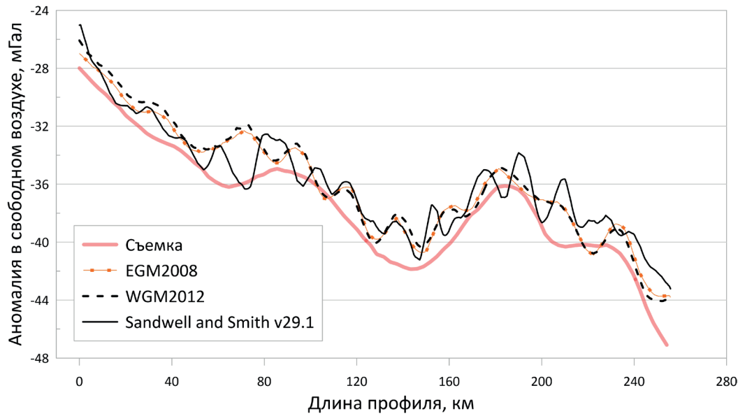
Рис. 7. Графики данных морской гравиметрической съемки и моделей ГПЗ в абиссальной области (Индийский океан)
