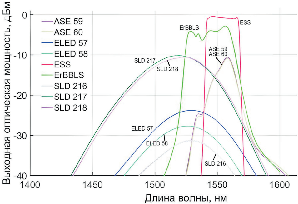
Рис. 2. Спектры оптического излучения нескольких источников при комнатной температуре и паспортном значении тока накачки (здесь для наглядности оптическая мощность выражена в дБм)
