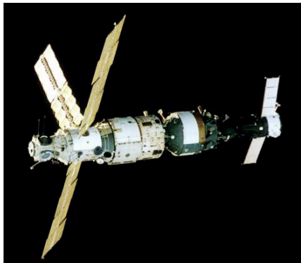
Рис. 6. ОК «Мир» в 1987 г. (базовый блок, модуль «Квант» и корабль «Союз-ТМ»)
