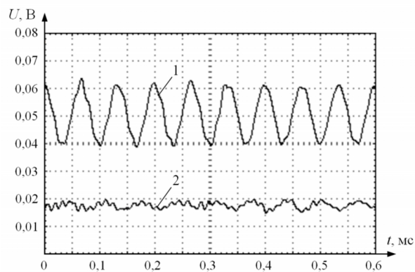
Рис. 4. Осциллограмма: 1 – сигнал с датчика угла гироскопа Д-7; 2 – сигнал с датчика угла модернизированного гироскопа
