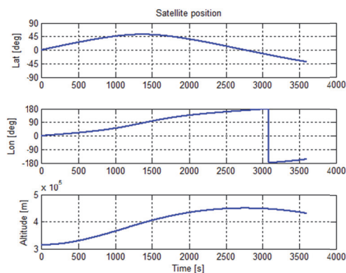
Рис. 6. Орбита МКС
